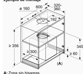
Dimensiones en mm Ejemplo de montaje
