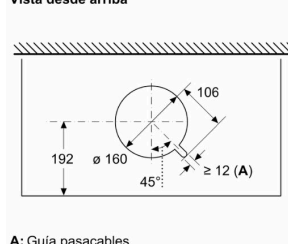
Dimensiones en mm Vista desde arriba
