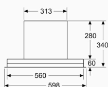
Dimensiones en mm Vista frontal
